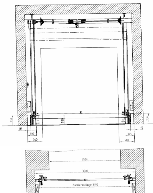
Plan de montage: modèle IBS-BHV
