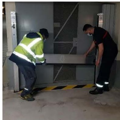
Exercice d'installation d'un batardeau © PariSeine
