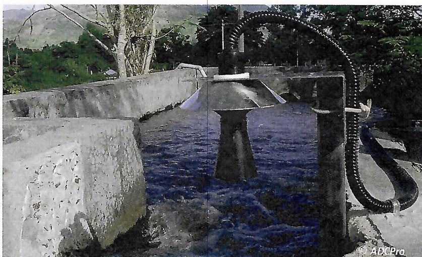
Le choix d'une solution dépend d'abord de la largeur, du marnage, de la profondeur d'eau, ou encore de la morphologie du terrain, chaque technologie (ici, un capteur de niveau à ultrasons Mach U) ayant ses avantages et ses limites.
